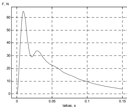
5 pav. Variklio jėgos dinaminė charakteristika, gauta modeliuojant variklį \alpha, \beta koordinaciu sistema
