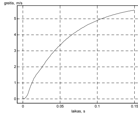
6 pav. Variklio greičio dinaminė charakteristika ( \alpha, \beta - koordinaciu sistema)
