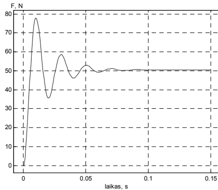
8 pav. Sustabdyto variklio jėgos dinaminė charakteristika ( \alpha, \beta koordinaciu sistema)
