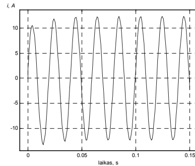
7 pav. Induktoriaus srovės dinaminė charakteristika \alpha, \beta koordinaciu sistema
