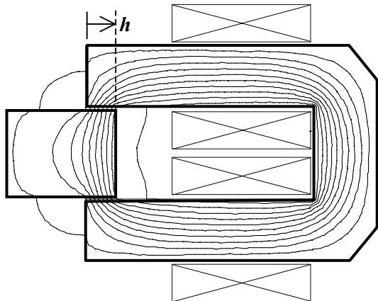
1 pav. Švytuojamojo sinchroninio variklio magnetinės dalies schema ir magnetinio lauko vaizdas
