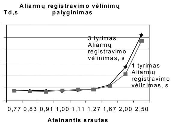
8 pav. Modeliuojamos apsaugos sistemos aliarmų registravimo vėlimo charakteristikų palyginimas
