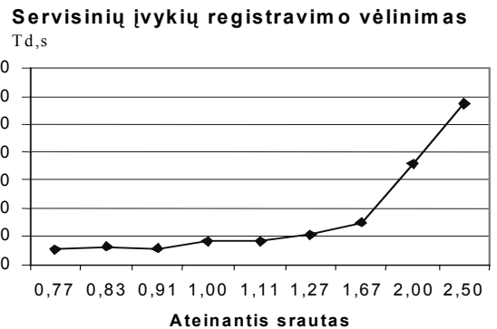
7 pav. Modeliuojamos apsaugos sistemos servisinių įvykių registravimo vėlimo charakteristika
