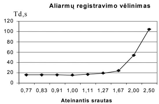
6 pav. Modeliuojamos apsaugos sistemos aliarmų registravimo vėlimo charakteristika
