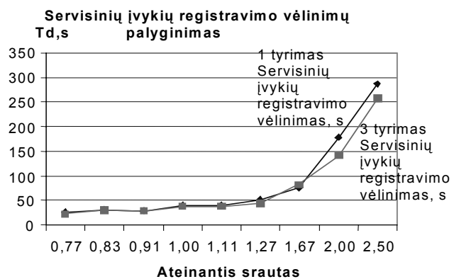
9 pav. Modeliuojamos apsaugos sistemos servisinių įvykių registravimo vėlimo charakteristikų palyginimas
