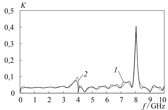
13 pav. Perdavimo koeficientų iš spiralės į bendraašės linijos prievadus, apkrautus varžomis Z_{e1} ir Z_{e2} , dažninės priklausomybės sistemoje su 35,5 mm ilgio bendraaše linija: 1 – tiesioginės bangos; 2 – atbulinės bangos
