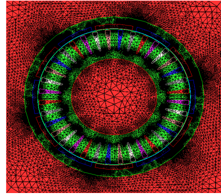
Fig. 5. Mesh production
