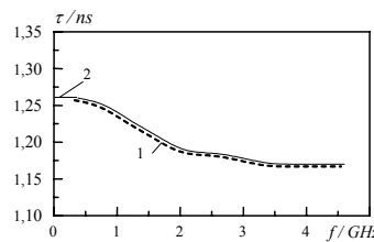
7 pav. Fazinio vėlinimo trukmės dažnines priklausomybės apskaičiuotos: 1 – pagal (4) formulę, 2 – pagal (6) formulę
