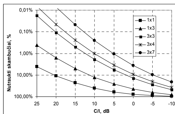
2 pav. Skambučių nutrūkimo priklausomybė nuo trukdžių. Čia 1x1, 1x3, 3x3, 3x4, 3x7 yra pakartotinio naudojimo schemos kai dažniai pakartotinai naudojami kas 1, 3, 9, 12 ir 21 narvelį
