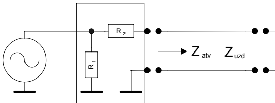
2 pav. Linijos pilnutinės varžos nustatymas
