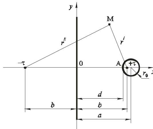
2 pav. Elektrodų sistema „laidas šalia plokštumos“
