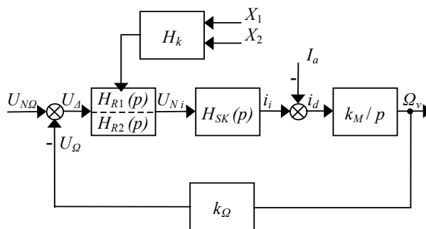
1 pav. Greičio reguliavimo kontūro su automatiškai keičiamos struktūros reguliatoriumi struktūrinė schema
