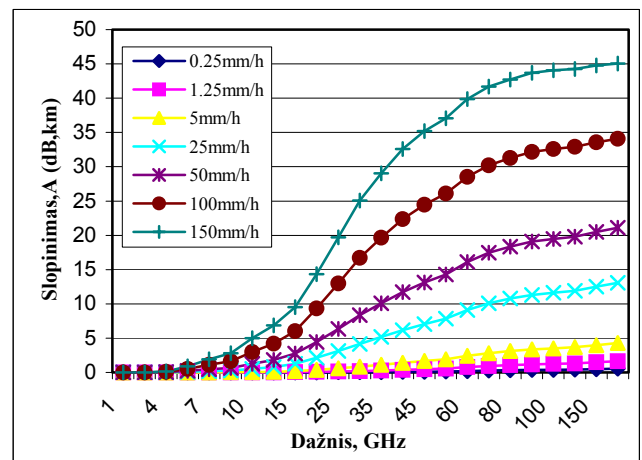
2 pav. Lietaus sukeliamas signalo slopinimas (signalų poliarizacija vertikali, lietaus temperatūra – +20° C)
