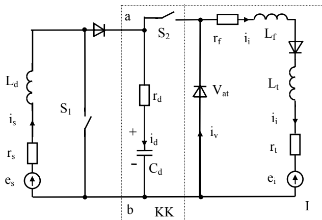
1 pav. Keitiklio ekvivalentinė schema
