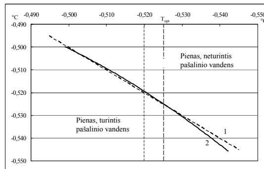
8 pav. Užšalimo temperatūros priklausomybė nuo specifinio elektrinio laidumo atlikus perskaičiavimą pagal (2) lygtį
