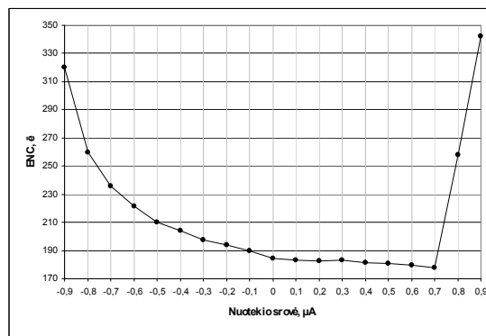
10 pav. Ekvivalentinio triukšmų krūvio priklausomybė nuo nuotėkio srovės ( Q_{in}=10 fC, C_d=0,2 pF, R_L=1 M \Omega , C_L=2,5 pF, T_{ap}=+27 °C)
