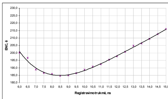
9 pav. Ekvivalentinio triukšmo krūvio ENC priklausomybė nuo registravimo trukmės ( Q_{IN}=10 fC, C_d=0,2 pF, R_L=1 M \Omega , C_L=2,5 pF)
