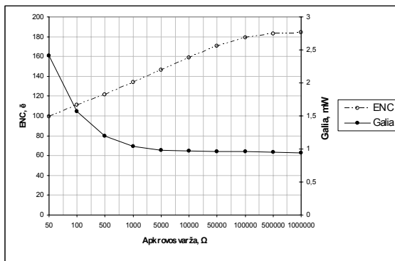
8 pav. ENC ir vartojamosios galios priklausomybė nuo apkrovos varžos ( C_d=0,2 pF, Q_{in}=10 fC, C_L=2,5 pF, išskyrus 50 \Omega apkrovą, kai C_L=0 pF, T_{ap}=+27 °C)
