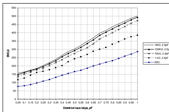
11 pav. ENC priklausomybė nuo jutiklio talpos, esant įvairioms KJS apkrovoms ( Q_{in}=10 fC, T_{ap}=+27 °C)
