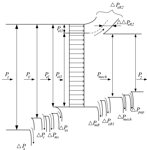
1 pav. Grežinių tyrimo mechatroninių įtaisų nesimetrinio asinchroninio elektros variklio galių diagrama
