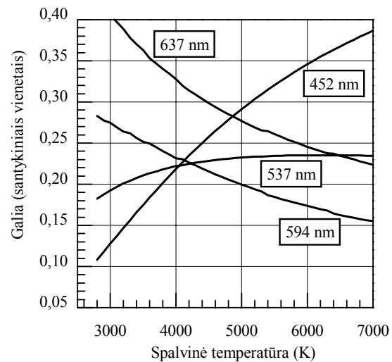
1 pav. Pirminių spinduolių srautų galių priklausomybės nuo šaltinio spalvinės temperatūros grafikai. Prie grafikų nurodyti PS grupių GSP funkcijų smailių bangos ilgiai
