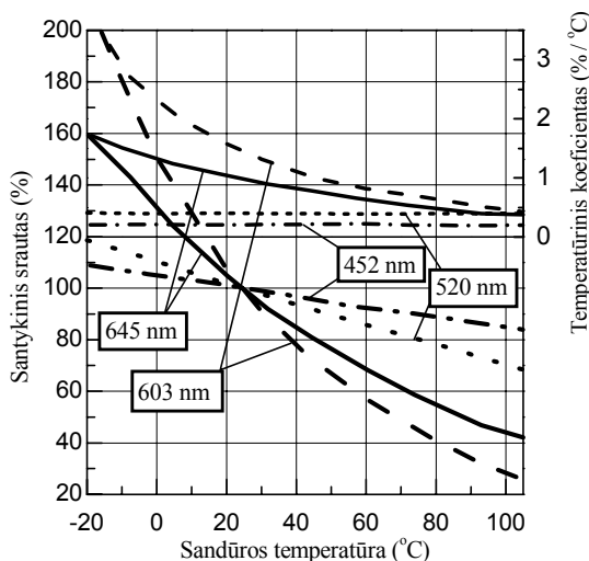
2 pav. Spindulių santykinio srauto (apatinės kreivės) ir jų temperatūrinių koeficientų absoliučių verčių (viršutinės kreivės) priklausomybės nuo sandūros temperatūros grafikai. Prie grafikų nurodyti PS GSP funkcijų smailių bangos ilgiai
